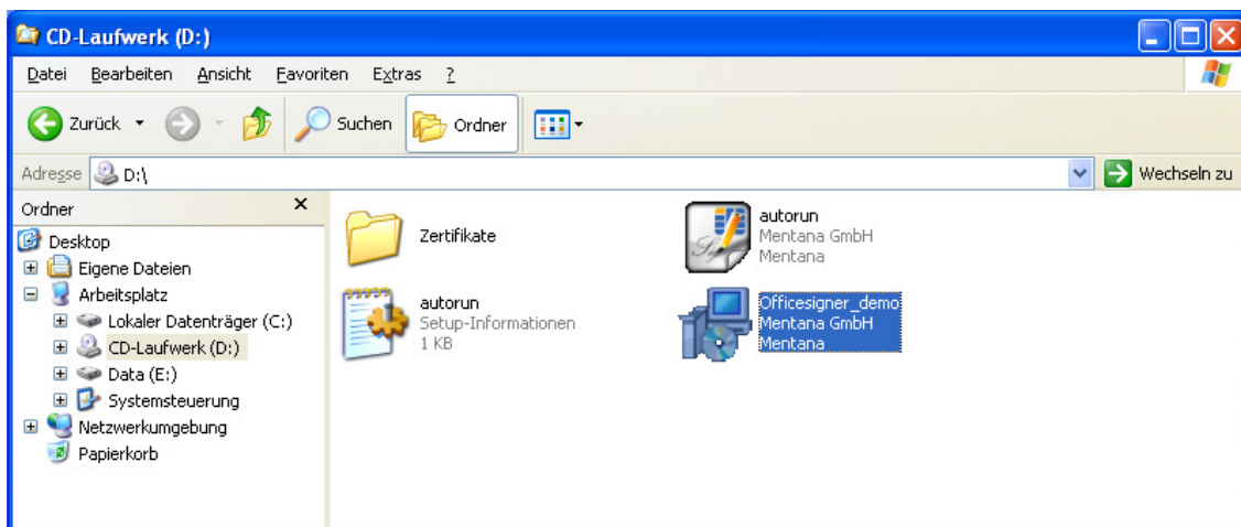
Abbildung 0-1 – Setup
