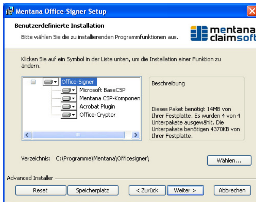
Abbildung 0-5 – Komponenten auswählen
