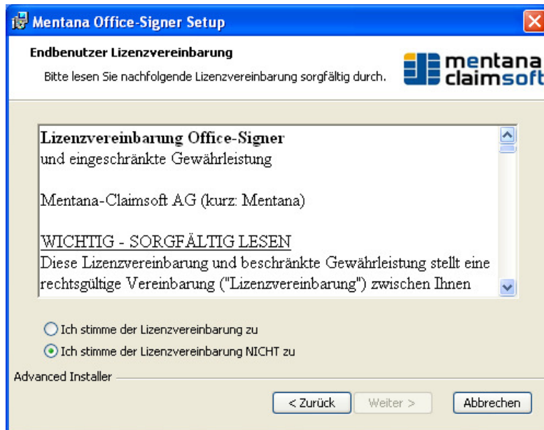
Abbildung 0-3 – Lizenzbedingungen
