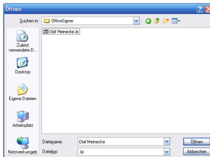
Abbildung 0-10 – Lizenz-Datei öffnen
