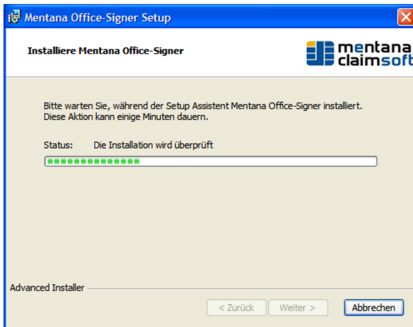
Abbildung 0-7 Installationsverlauf
